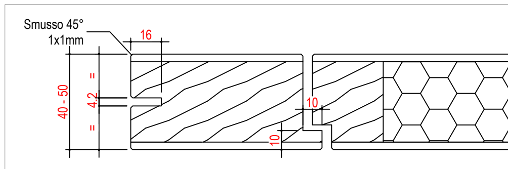
Dettaglio Sez. B
