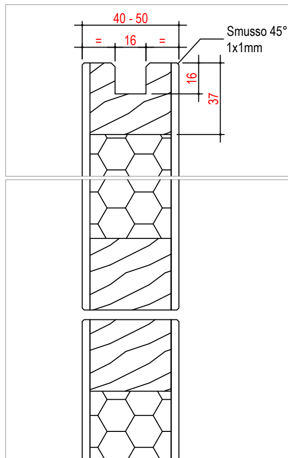
Dettaglio Sez. A
